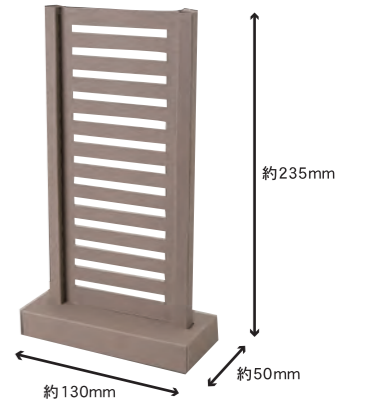
T90A2 ミニチュア パーテーション
